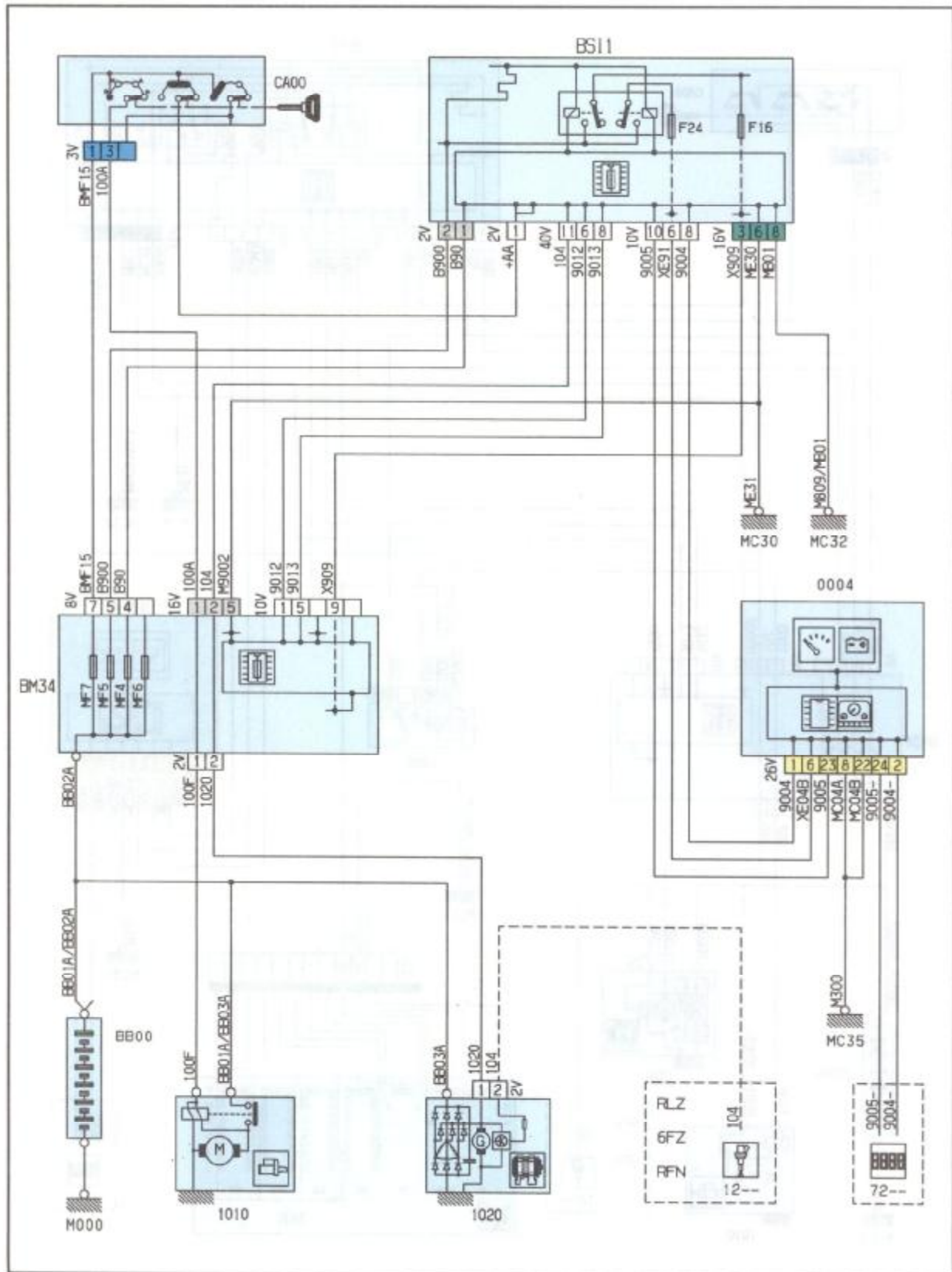
Схема 7. Стартер. Автомобили с бензиновым двигателем EW7J4 (6FZ)/EW10J4 (RFN)/EW10D (RLZ) и механической коробкой переключения передач
