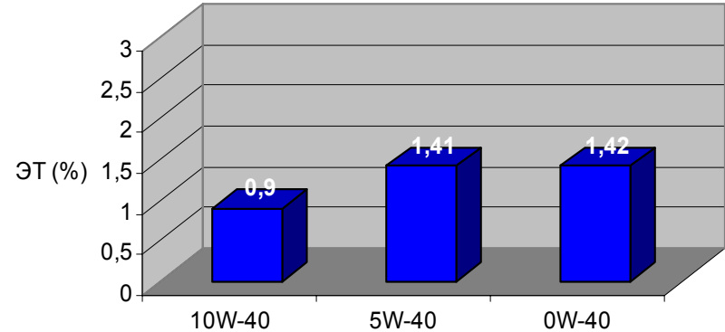
Экономия топлива при низких температурных режимах
