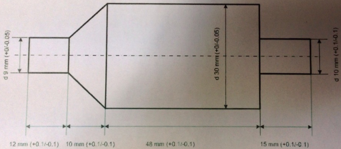
Стопор КВ
