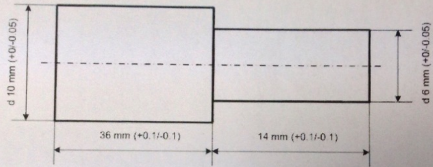
Стопор РВ
